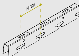
Carrier TR2
