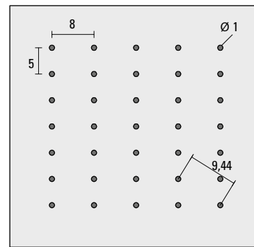
Foratura lineare FL01
