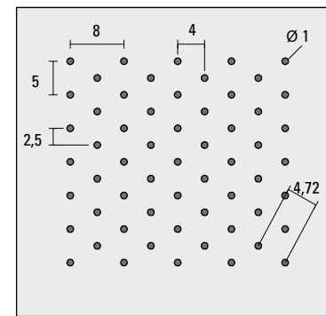
Foratura diagonale FD01
