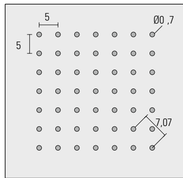
Foratura lineare FL00,7
