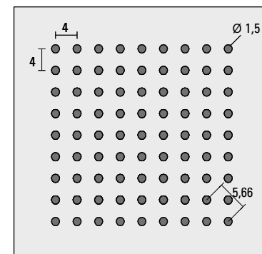
Foratura lineare FL01,5
