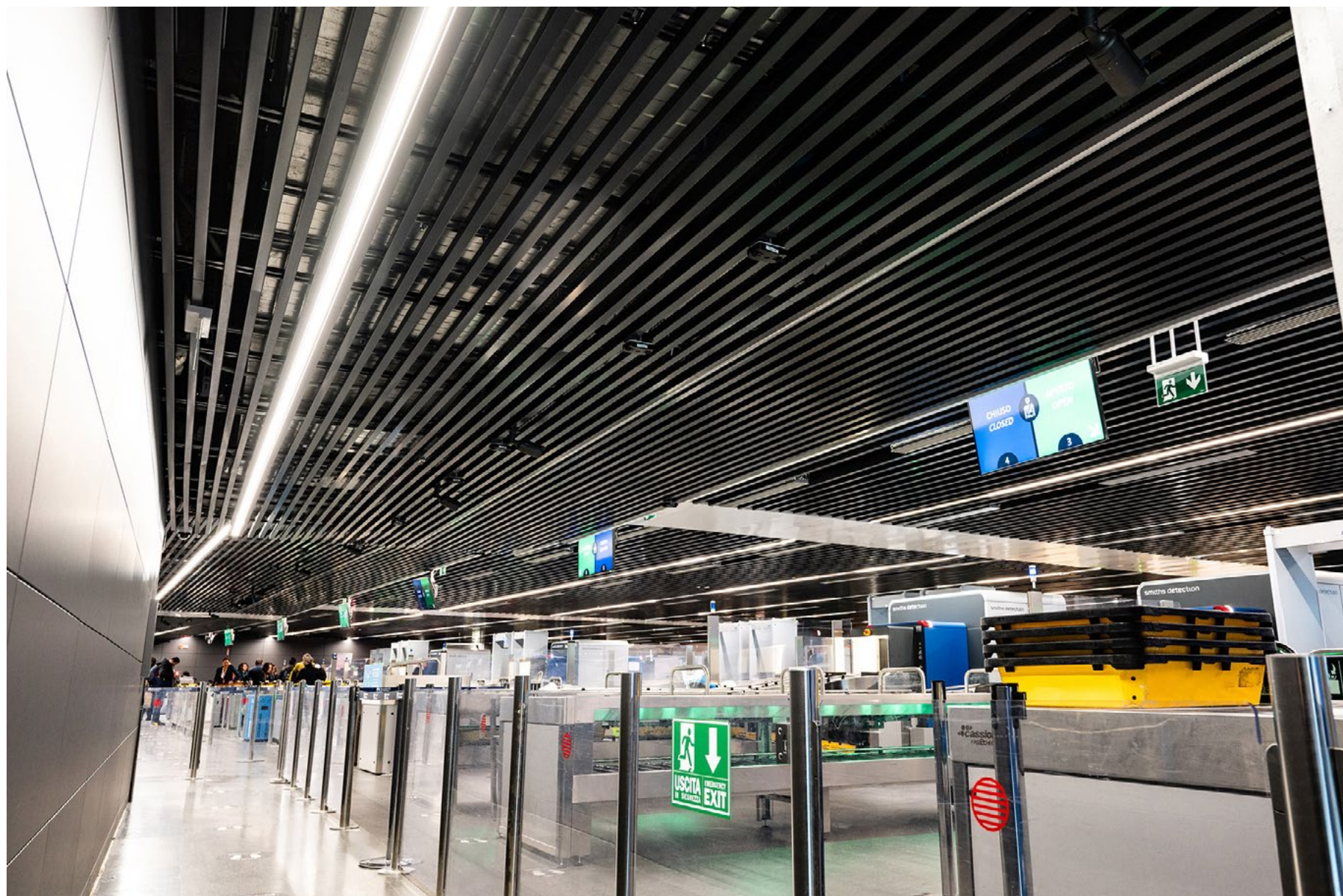
Doghe Q-Baffle , colore RAL 7016 opaco, acciaio zincato (DX51DZ), base liscia con microforatura sui lati.
