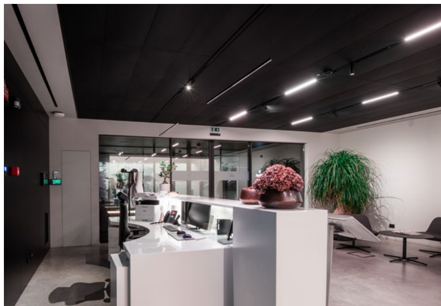
Vert Occulto 600x1200 mm in acciaio zincato e finitura post-verniciata, con foratura Ø2mm e velo di tessuto non tessuto per incremento del comfort acustico.
