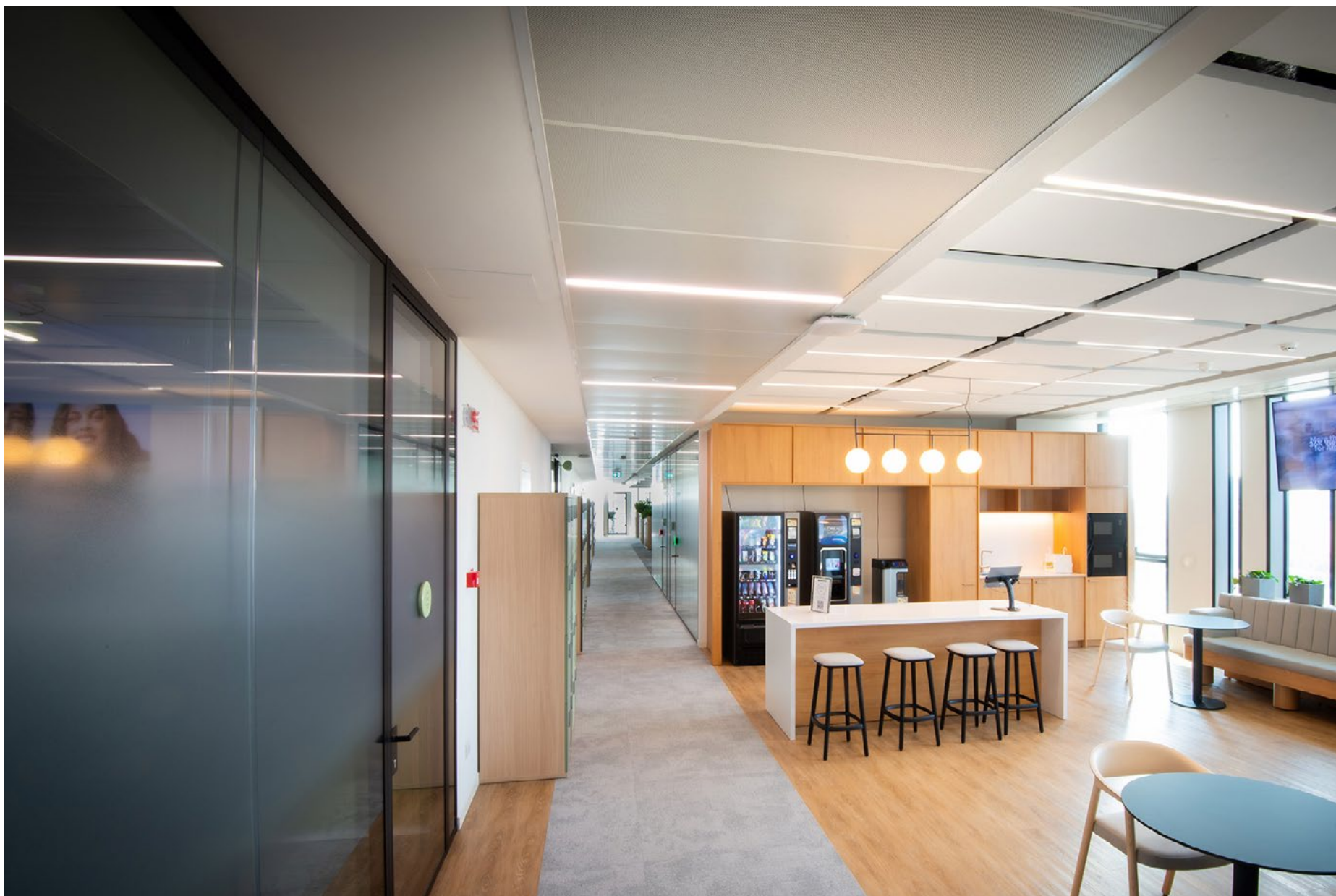
Pannelli autoportanti tipo "C" e "Q" con dimensioni variabili, foratura Ø2mm e velo di tessuto non tessuto per incremento del comfort acustico.
