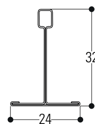
Section: IL 1200 mm IC 600 mm
