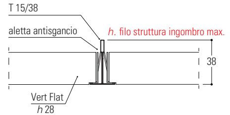
Sistema con plenum
