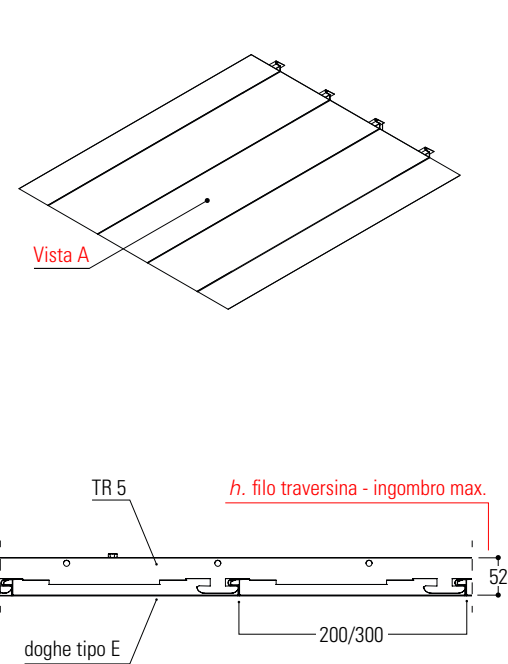
Sistema con doghe tipo "E"
