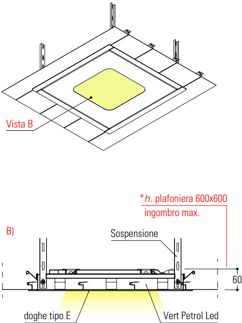
Sistema con doghe tipo "E" con plafoniera
