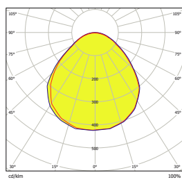
Vert Reticula Led 200 64W UGR
