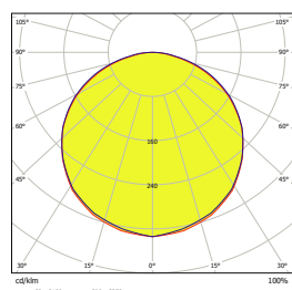
Vert Reticula Led 200 64W OP
