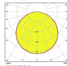
Vert Reticula Led 144 45W OP
