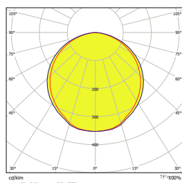
Vert Reticula Led 84 32W OP
