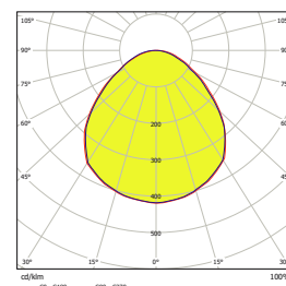
Vert Reticula Led 265 70W UGR
