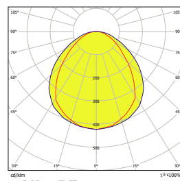
Vert Reticula Led 192 70W UGR
