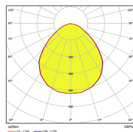
Vert Reticula Led 144 45W UGR
