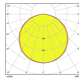
Vert Reticula Led 265 70W OP
