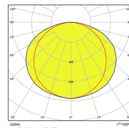
Vert Reticula Led 192 70W OP
