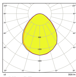
Vert Reticula Led 84 32W UGR
