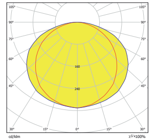
Vert Reticula 192 75W OP
