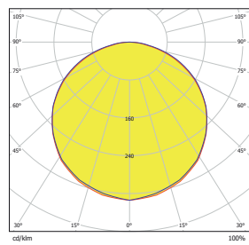
Vert Reticula 200 80 W OP
