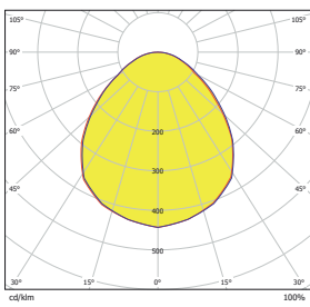
Vert Reticula 200 80 W UGR
