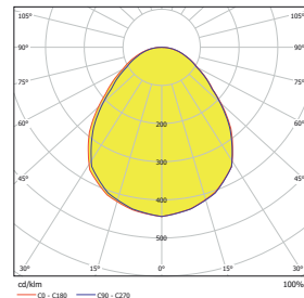
Vert Reticula 144 56W UGR
