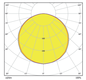
Vert Reticula 265 90 W OP
