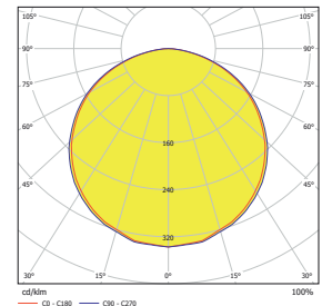
Vert Reticula 144 56W OP
