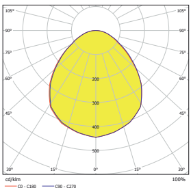
Vert Reticula 100 40 W UGR
