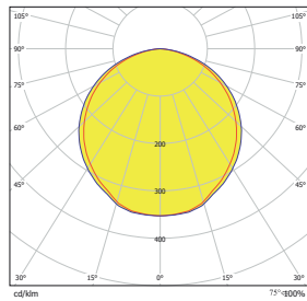
Vert Reticula 84 38W OP
