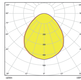
Vert Reticula 265 90 W UGR
