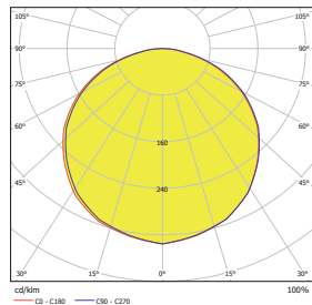
Vert Reticula 100 40 W OP
