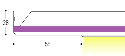
Beveled edge
